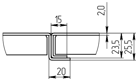
ВИД А 1 : 2
